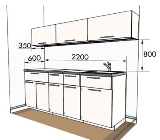
Варианты стандартных размеров кухни
