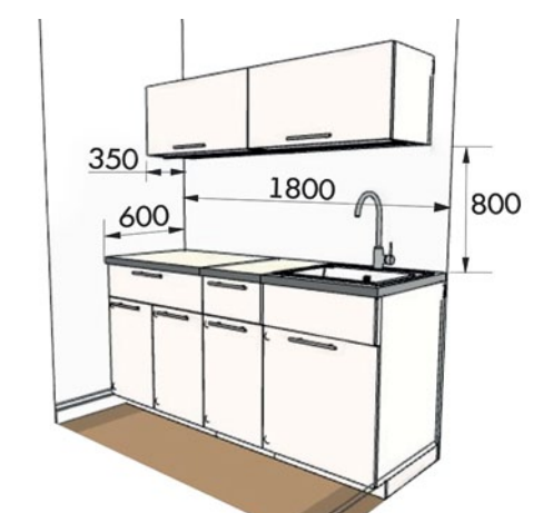
Варианты стандартных размеров кухни
